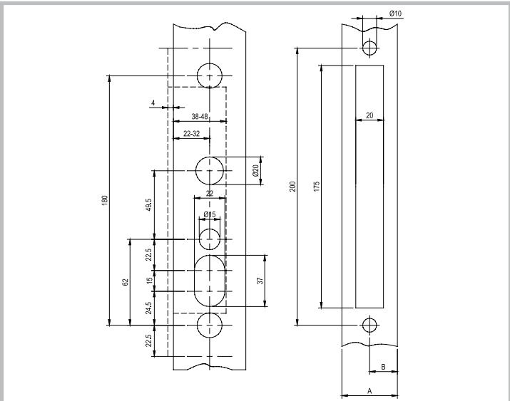
Lock case 5016: aluminium door
